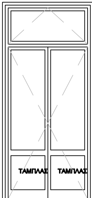
ΔΙΦΥΛΛΑ ΑΝΟΙΓΟΜΕΝΑ ΥΑΛΟΣΤΑΣΙΑ ΕΞΩΣΤΟΘΥΡΩΝ ΠΡΟΣΟΨΗΣ
